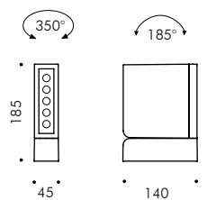
KEEN 5 LED Ø 140
