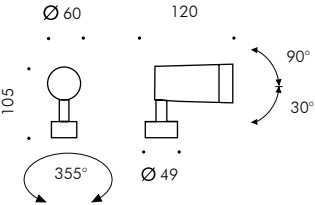
FLOWER ZOOM Ø60 PROIETTORE Flower ZOOM Ø60 spotlight
