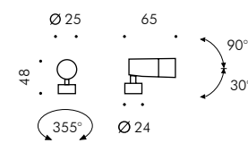
FLOWER Ø25 PROIETTORE Flower Ø25 spotlight
