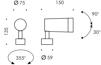
FLOWER ZOOM Ø75 PROIETTORE Flower ZOOM Ø75 spotlight
