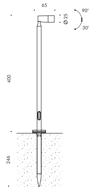
FLOWER Ø25 PICCHETTO H400 Flower Ø25 garden spike H400
