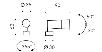
FLOWER Ø35 PROIETTORE Flower Ø35 spotlight
