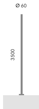
S.2843 PALO CILINDRICO Ø 60 mm FLANGIATO Altezza totale del palo 3500 mm
