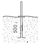
S.2806 ACCESSORIO FLANGIA DA INTERRARE Altezza totale 1000mm Da interrare per una profondità di 500mm
