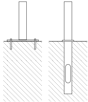
MANDATORY ACCESSORIES FOR MINISHIFT POLE INSTALLATION TO BE CHOOSEN BETWEEN Accessoires obligatoires pour l'installation sur mât de Minishift au choix entre
